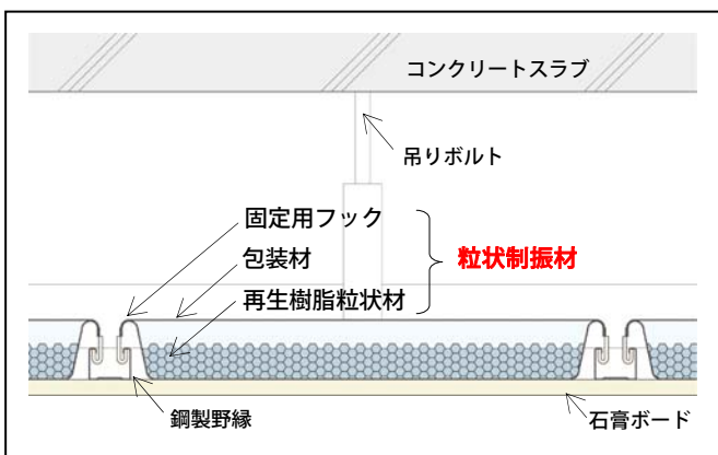
図1 天井断面詳細図
