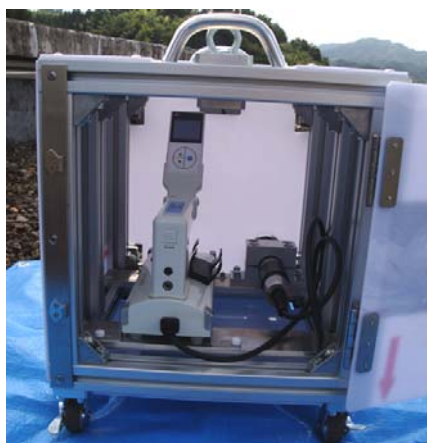
写真3 「さー兵衛」測定装置内部
