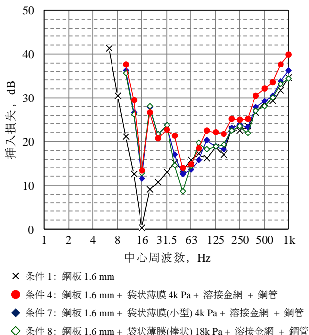
図-13 袋状薄膜の形状と挿入損失の関係
