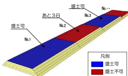
② 盛土速度の見える化システム (施工管理の省力化・効率化)
